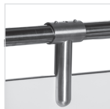
Horný trubkový profil, priemer 30 mm (nerez), do šírky dosky 60 mm nemusí byť horný profil použitý
